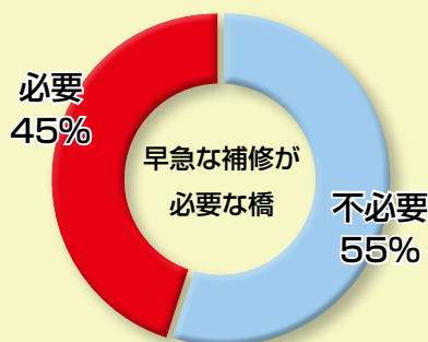
橋齢 40 年以上の直轄国道の 橋梁の点検結果 (平成 19 年 国土交通省調べ)
